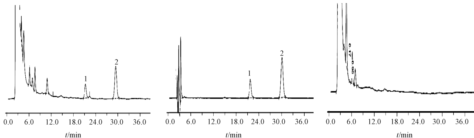
图 1 大黄素、大黄酚 HPLC 图
